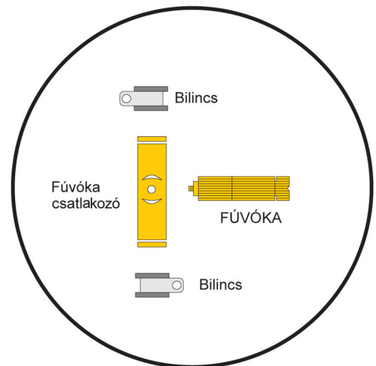
Összeállítási Rajz
